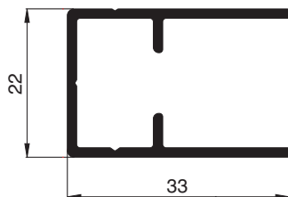
10 45 04 Rahmenprofil
