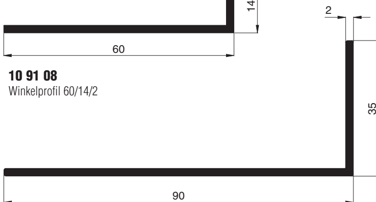
10 91 30 Winkelprofil 90/35/2
