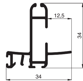
10 39 20 Gewebeschiene für Blendrahmenabdichtung innen
