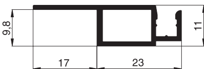
10 23 09 Spannrahmenprofil
