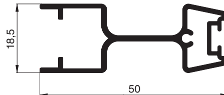
10 45 05 Griffleiste
