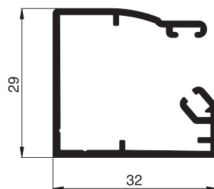
10 40 05 seitliche Führungsschiene
