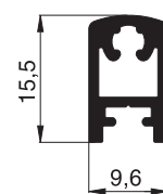
10 39 21 unteres Rahmenprofil
