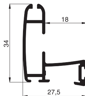
10 39 18 Gewebeschiene für Blendrahmenabdichtung
