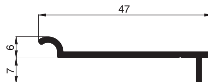
10 43 13 Kastenblende unten
