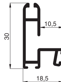
10 40 08 Gewebeschiene
