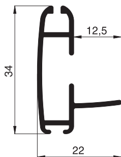
10 39 17 Gewebeschiene
