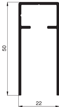
10 45 02 Kastenprofil 50 mm
