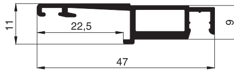
10 22 04 Spannrahmenprofil
