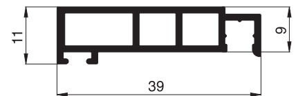
10 24 52 Spannrahmenprofil
