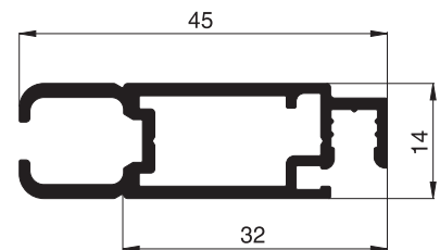
10 34 07 Pendeltürprofil
