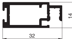
10 34 06 Pendeltürprofil
