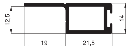
10 34 28 Montagerahmenprofil
