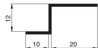
10 26 07 Z-Schiene
