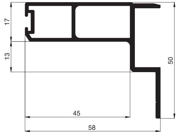
10 32 16 Lichtschachtabdeckungsprofil
