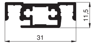
10 36 11 Sprossenprofil
