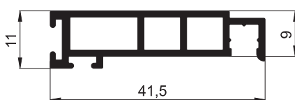
10 24 56 Spannrahmenprofil
