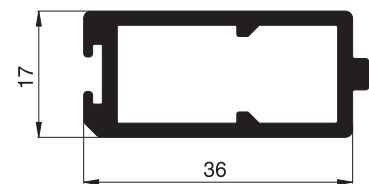
10 32 40 Adapterprofil
